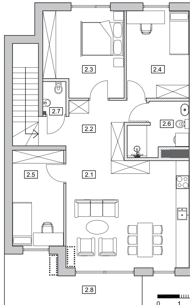
RZUT 2 PIĘTRA
